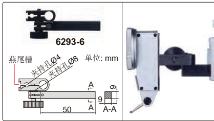
杠杆表支架(选配), 适用于1250-300/450/600
