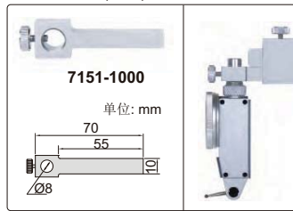
杠杆表支架(选配), 适用于1250-1000
